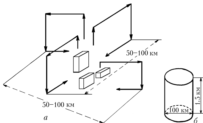
Схема образования локальной циркуляции вокруг города (а); схема расчетной области, принятая в настоящей работе (б)
